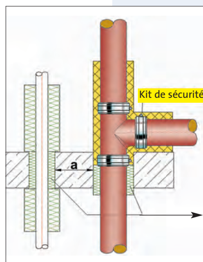
Fig. 2 : PAM-GLOBAL® pourvu de kit de sécurité incendie à côté de conduites protégées contre l'incendie, par ex. de la société Rockwool avec de l'ABP ou avec d'autres systèmes de sécurité incendie, par ex. avec des manchettes de sécurité incendie avec de l'ABZ.
